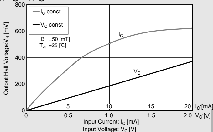
V_H-V_C, V_H-I_C
