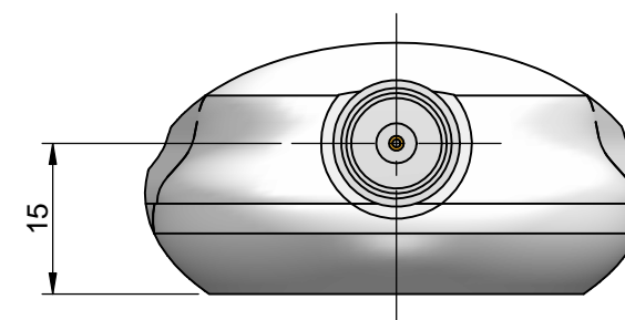
TNC CONNECTOR GIGATRONIX TN62-X001-N06
