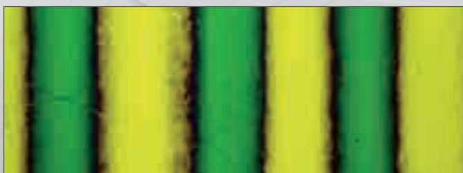
Abbildungen: Visualisierung der magnetischen Struktur von Linearencodern
